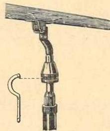
Ansicht der Klemmvorrichtung mit Schlüssel zu No. 16 b
