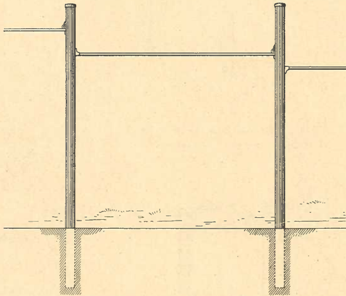
No. 33 a. Reck mit Pfosten aus starken Eisenröhren zum Einbetonieren mit Aufritten
