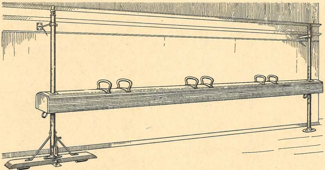
No. 30 a. Stemmbalken mit Rollständer, 3 Paar Pauschen
