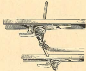
Roll- vorrichtung. Stellung der Rollen beim rollen
