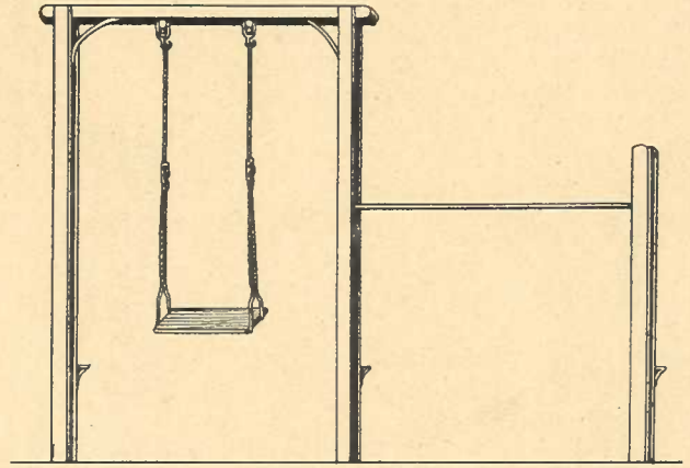
No. 83. Schaukelgerüst aus I-Balken, zum Einbetonieren mit Reck nebenan, mit beweglichen Haken
