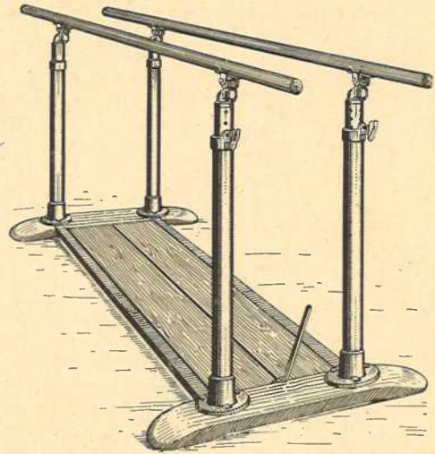
No. 16 a. Barren . Verstellung mit Federbolzen, Bodenbrett und Rollvorrichtung
