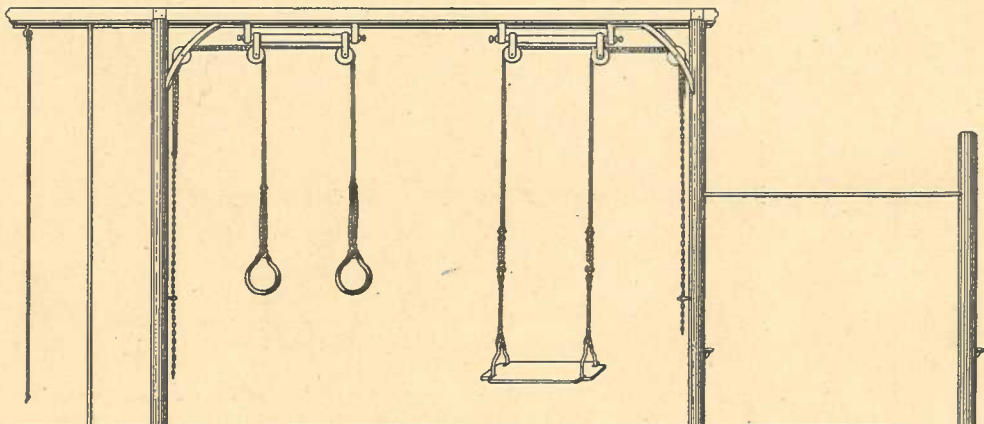
No. 87. Doppelttes Schaukelgerüst mit Reck, Kletterstange und Tau
