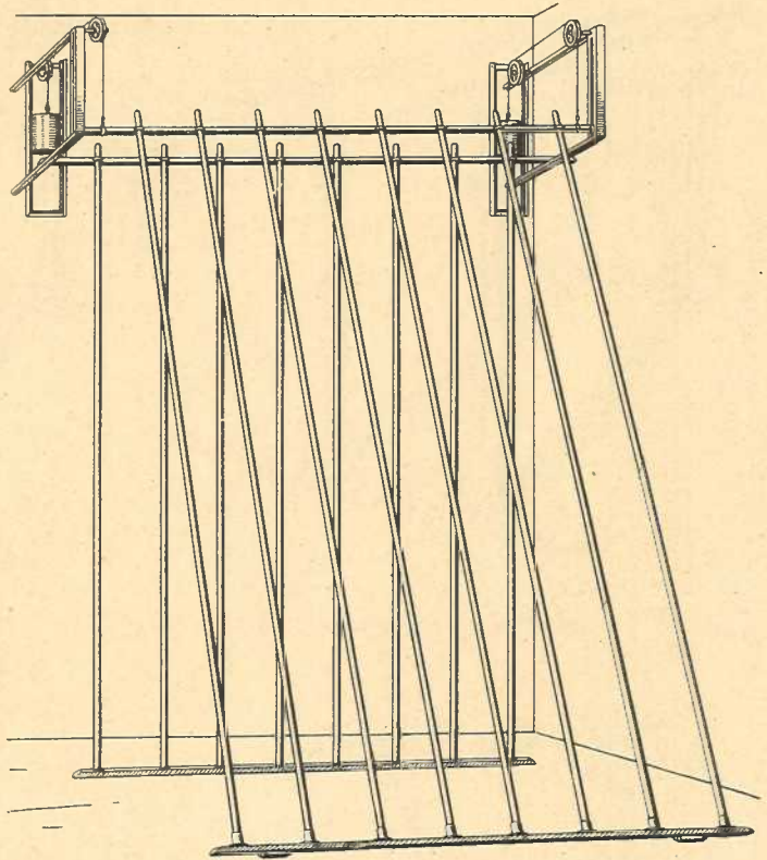
No. 62 a. Klettergerüst mit 16 Stangen in zwei Reihen, vordere Reihe mittelst Gegengewicht senkrecht und schräg verstellbar
