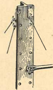
Spannreckständer mit Reckstangen- befestigung zu No. 36
