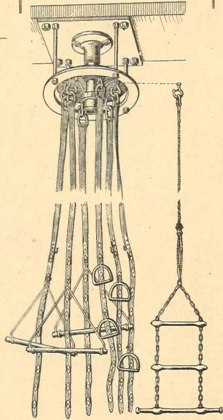
No. 49 c Rundlauf mit Schutzring und Kugellager, Lederriemen mit großen und kleinen Griffen
