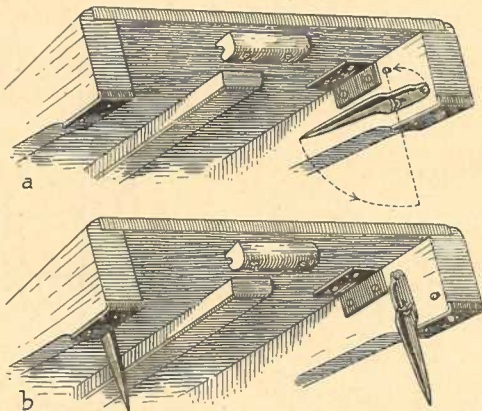
No. 44 c. Sprungbrett neue Façon mit Gummiplättli und umlegbaren Eisenspitzen
