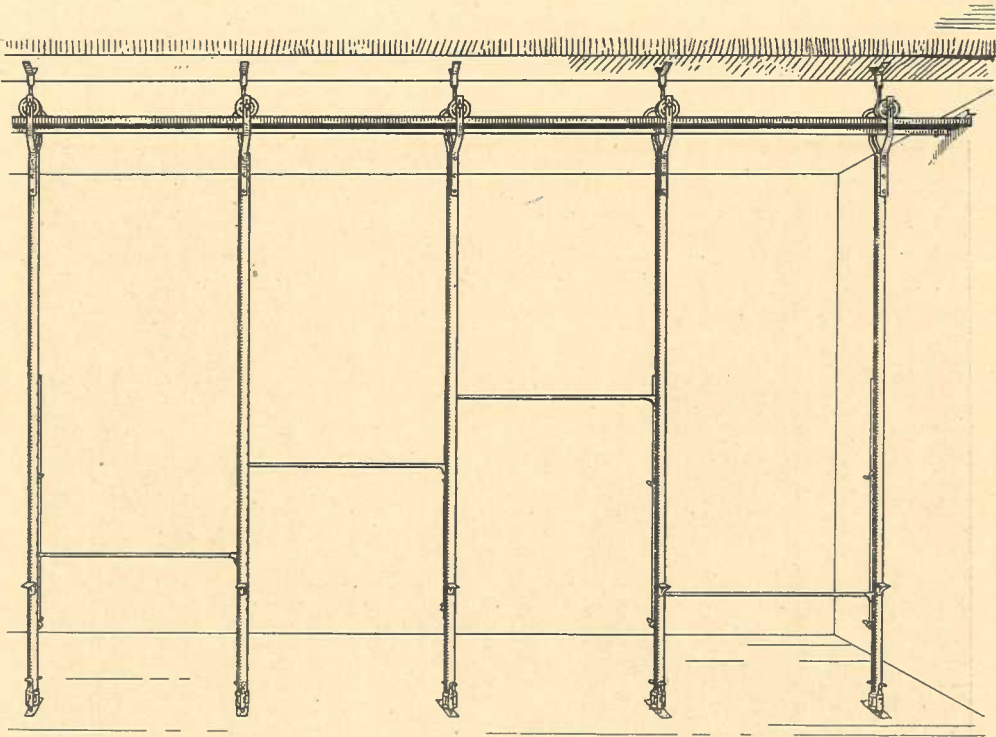
No. 40. Rollrecke mit Gleitschiene
