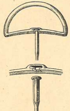
No. 26 b Bügelpausche mit Lederbezug, Griff und Stiften getrennt
