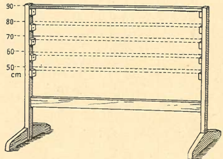
No. 72 a. Sprunghürde (Schulhürde) mit Latten 50-90 cm
