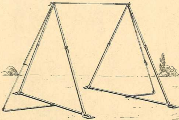
No. 37. Stellreck für Turnsaal und ins Freie
