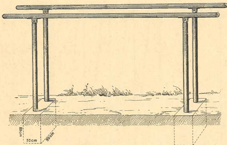
No. 3. Barren zum Einbetonieren, unverstellbar
