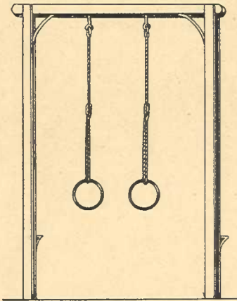
No. 81/82. Schaukelgerüst aus I-Balken zum Einbetonieren mit gewöhnlichen Haken, auch als Reck eingerichtet, in leichter und starker Ausführung
