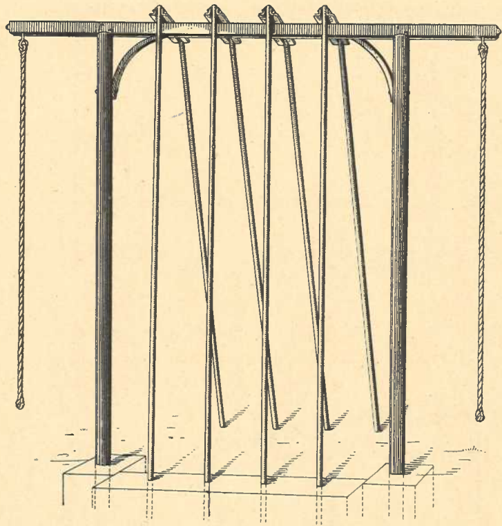
No. 60. Klettergerüst, Pfosten aus starken Eisenröhren zum Einbetonieren, 4 senkrechte u. 4 schräge Stangen und 2 Klettertaue
