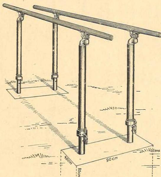
No. 7 a. Barren zum Einbetonieren hoch und weit verstellbar
